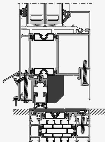
Nach außen öffnend Barrierefreie Nullschwelle
