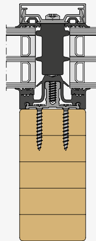
THERM + 50 H-I mit Dämmblock P
