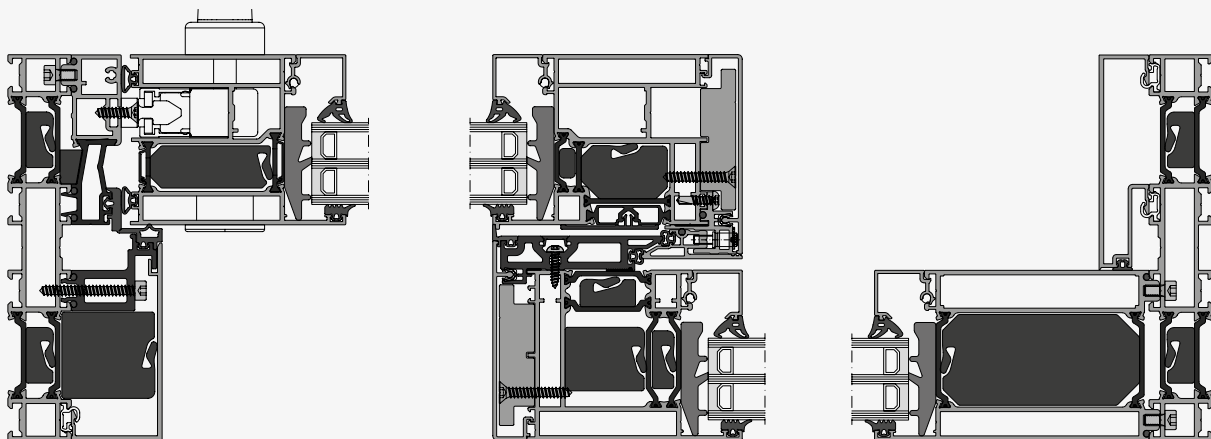
③ Hebe-Schiebeflügel
