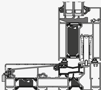
Hebe-Schiebeflügel Verglasung von innen (GI)
