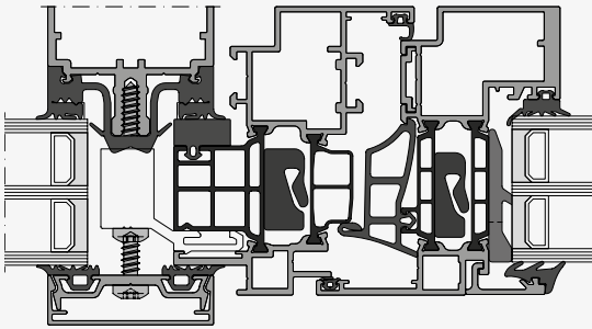
FRAME + 75 WA n. a. öffnend
