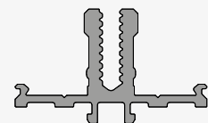
Grundprofil mit Fuß
