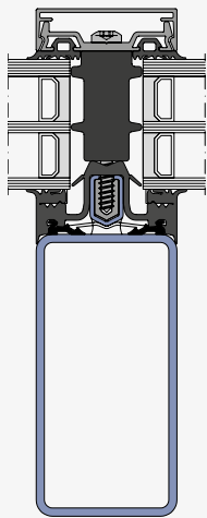
THERM + 50 S-I mit Dämmblock P
