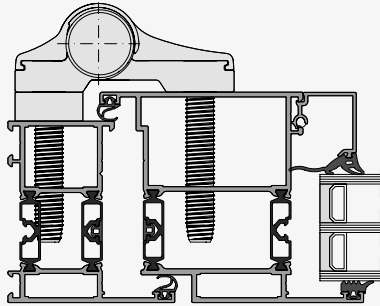
Aufschraubband n. i. 3-teilig mit Ankerschraube
