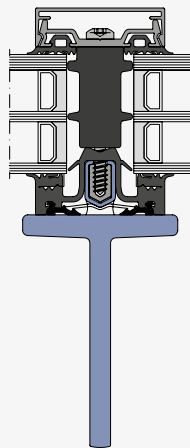
THERM + 50 S-I mit Dämmblock P und T-Tragprofil
