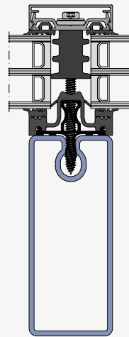
THERM + 50 FS-I mit Dämmblock P
