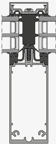
THERM + 50 A-I mit Dämmblock P
