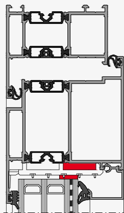
RC2 — Spezialglas zusätzliche Verklötzung + Verklebung
