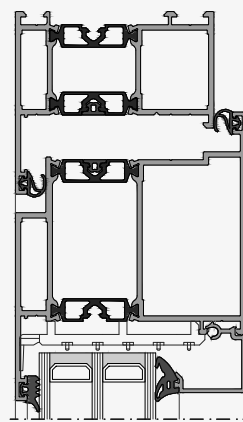
RC1N – Standardglas zusätzliche Verklötzung
