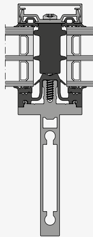
THERM + 50 A-I mit Dämmblock P und T-Tragprofil
