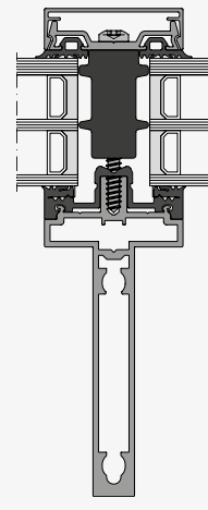
THERM + 50 A-V mit Dämmblock P und T-Tragprofil
