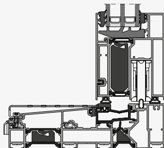
Hebe-Schiebeflügel Verglasung von außen (GO)
