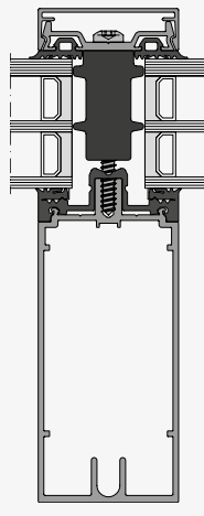
THERM + 50 A-V mit Dämmblock P
