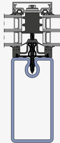
THERM + 56 FS-I mit Dämmblock P
