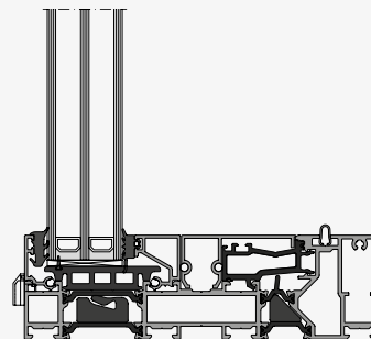
②.3 Direktverglasung von außen (GO)
