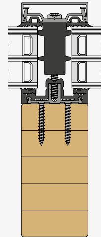
THERM + 50 H-V mit Dämmblock P
