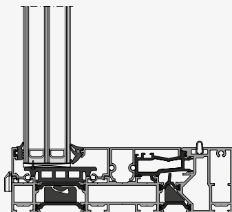
②.2 Direktverglasung von innen (GI)
