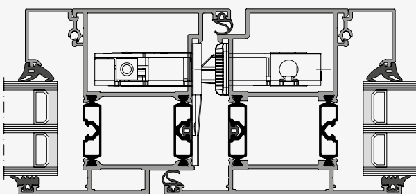
Paniktürschloss
