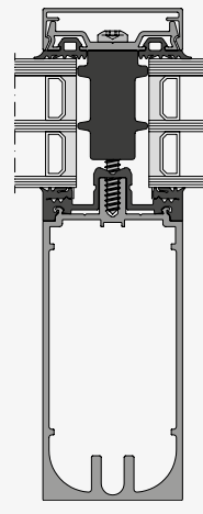
THERM + 50 A-V mit Dämmblock P und verstärktem Tragprofil
