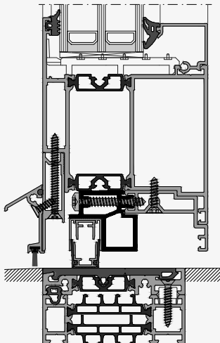
Nach innen öffnend Barrierefreie Nullschwelle
