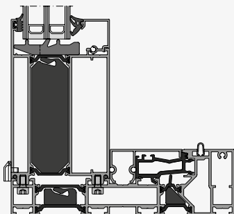
②.1 Festverglasungsprofil (GI)
