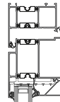
RC1N – Standardglas zusätzliche Verklötzung
