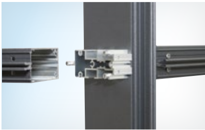
Pfosten-Riegel Verbinder
