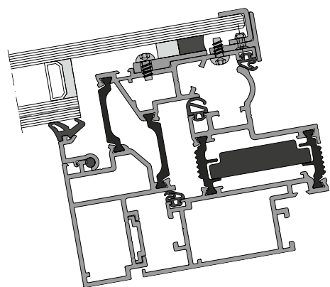
FRAME + 100 RI – Variante Stufenglas
