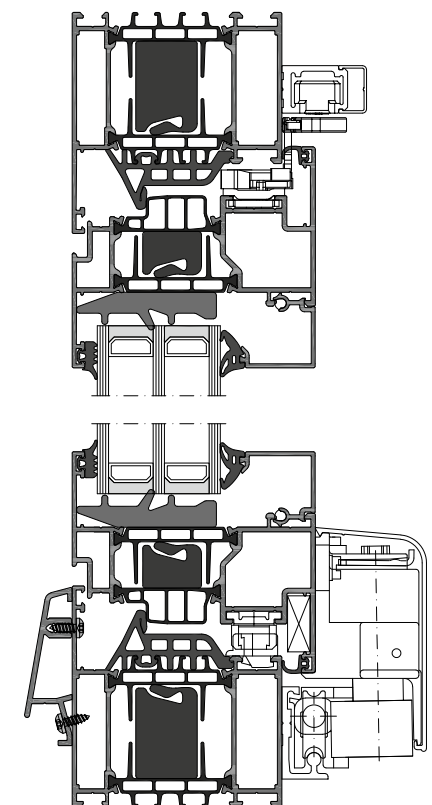
FRAME + 75 WI PSK
