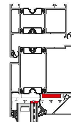
RC2 – Spezialglas zusätzliche Verklötzung + Verklebung
