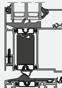
Mit Einschiebdämmung bis U_f
