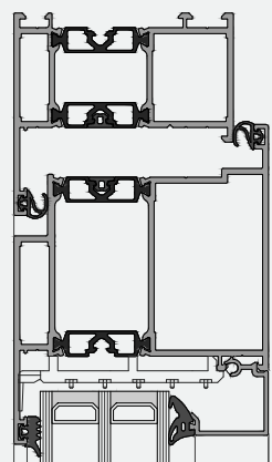
RC1N – Standardglas zusätzliche Verklotzung
