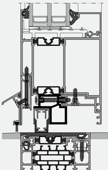
Nach innen öffnend Barrierefreie Nullschwelle
