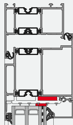
RC2 — Spezialglas zusätzliche Verklotzung + Verklebung
