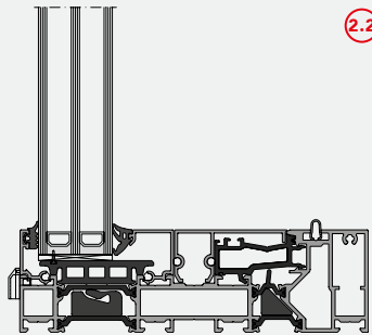
Direktverglasung von innen (GI)
