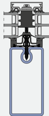
THERM + 56 FS-I mit Dämmblock P
