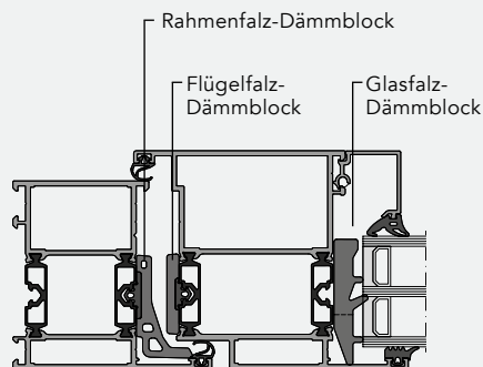
Ohne Einschiebdämmung bis U_f
