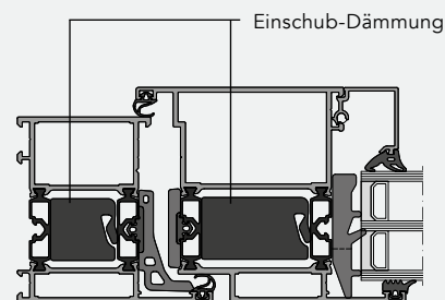
Mit Einschiebdämmung bis U_f
