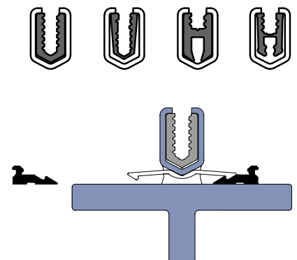
Abb. 1: Perfekter konstruktiver Korrosionsschutz
