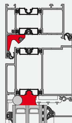
RC3 — Spezialglas, Falzverstärkung; zusätzliche Verklotzung + umlaufende Verklebung
