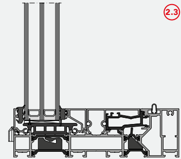
Direktverglasung von außen (GO)
