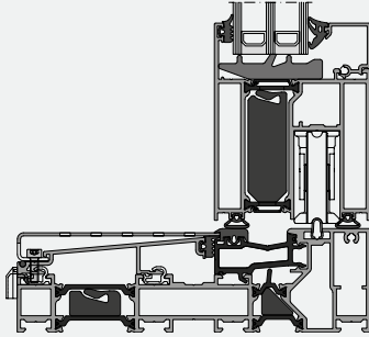
Hebe-Schiebeflügel Verglasung von innen (GI)
