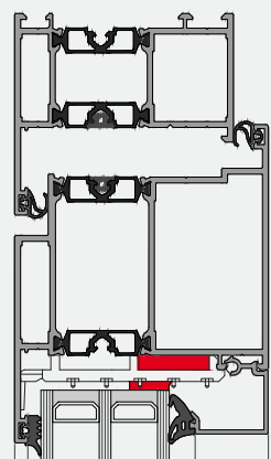
RC2N — Standardglas zusätzliche Verklotzung + Verklebung
