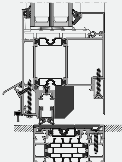
Nach außen öffnend Barrierefreie Nullschwelle
